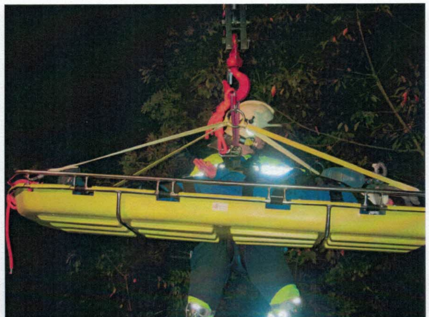
Der Schleifkorb eignet sich vor allem für Bergungen aus schwierigem Gelände. (Bild: Feuerwehr Zofingen)
